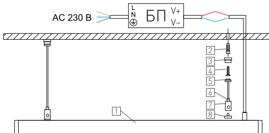
Рис. 2. Монтаж светильника
