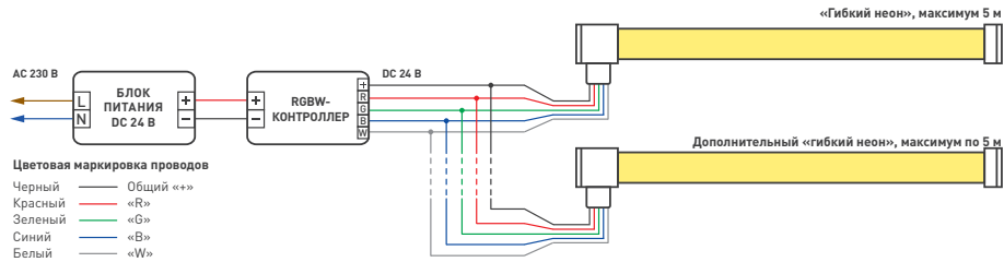
Схема 1. Подключение герметичной ленты «неон»
