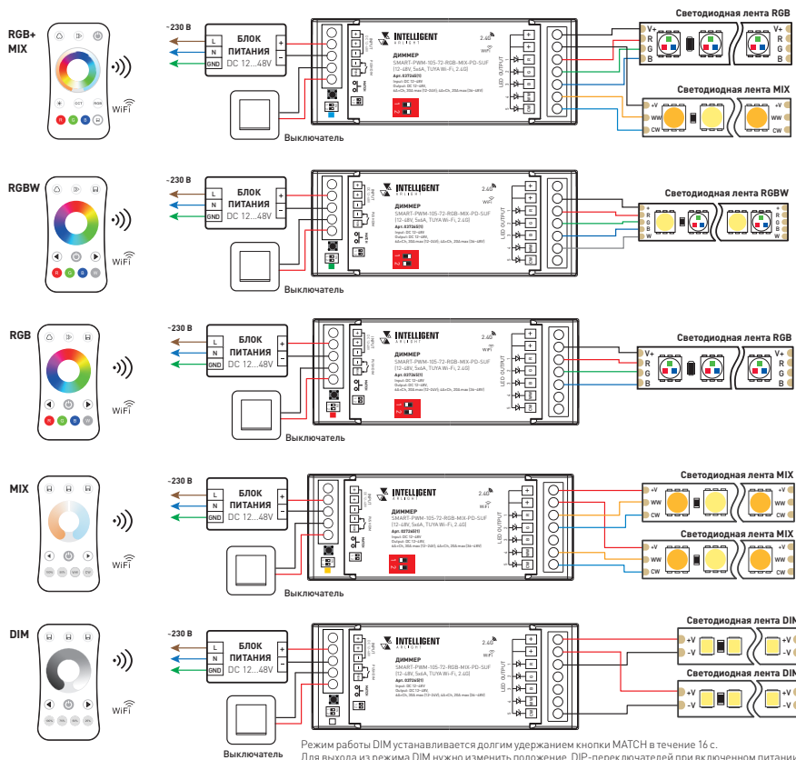
Рис. 1. Схемы подключения диммера SMART-PWM-105-72-RGB-MIX-PD-SUF
