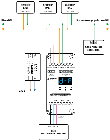
Рис. 3. Схема подключения при конвертации DMX в DALI
